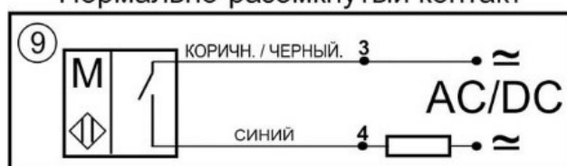
Схема соединения
