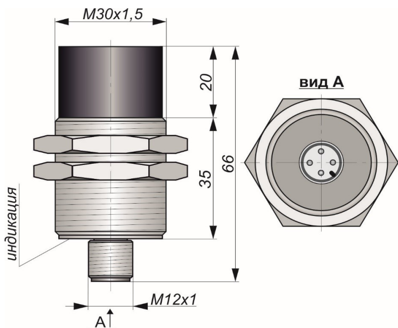
Габаритный чертеж
