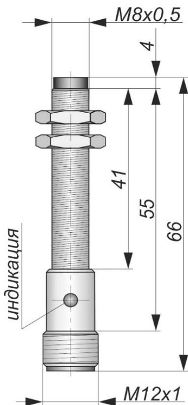
Габаритный чертеж
