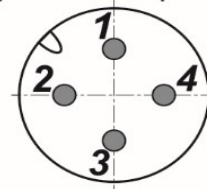
Цоколевка разъема
