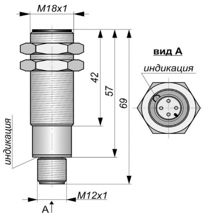
Габаритный чертеж
