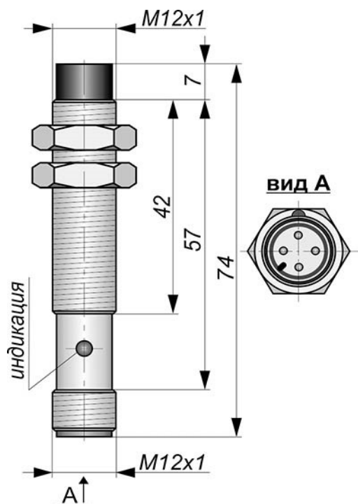
Габаритный чертеж
