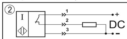
Цоколевка разъема
