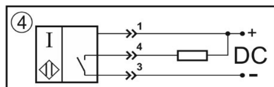
Схема соединения Нормально-разомкнутый контакт
