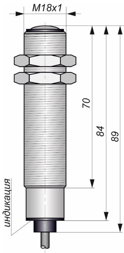
Габаритный чертеж
