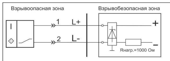
Цоколевка разъема
