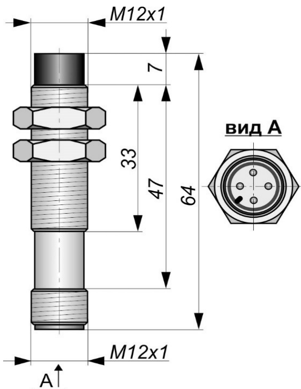
Габаритный чертеж
