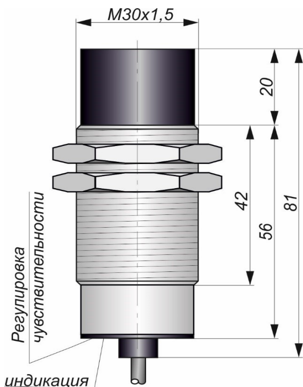
Габаритный чертеж
