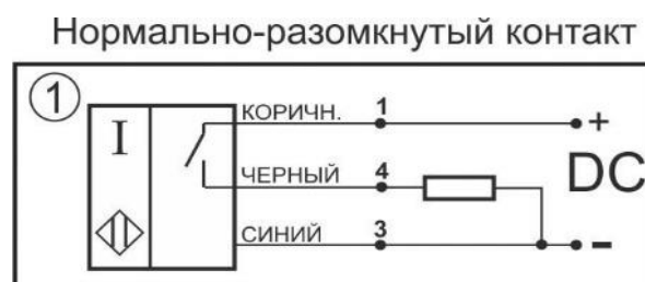
Цоколевка разъема
