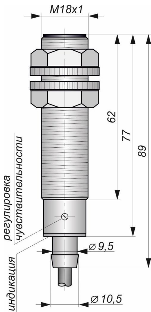
Габаритный чертеж
