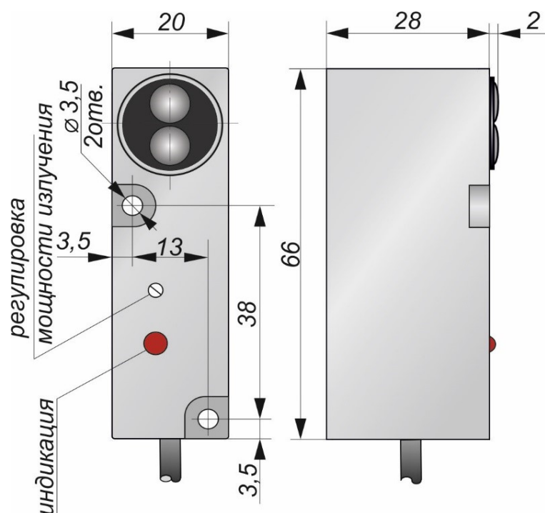
Габаритный чертеж
