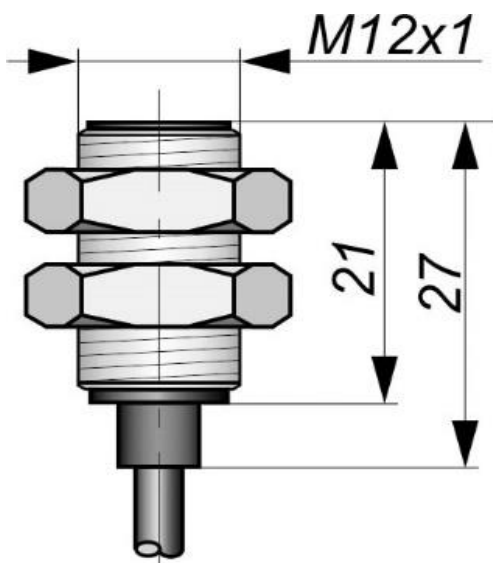
Габаритный чертеж
