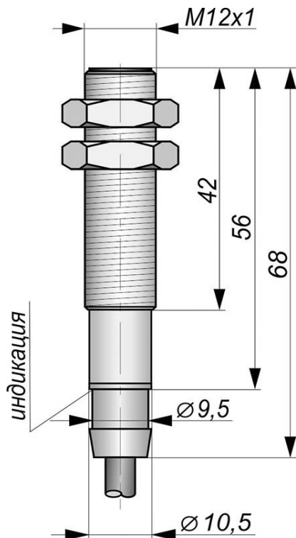
Габаритный чертеж
