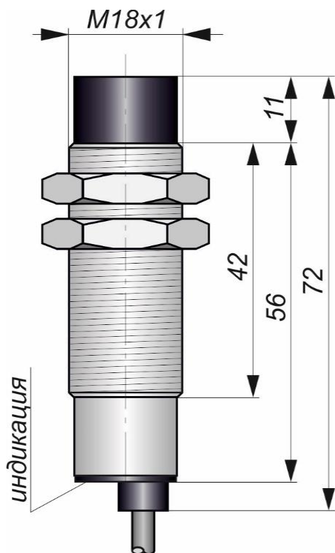
Габаритный чертеж
