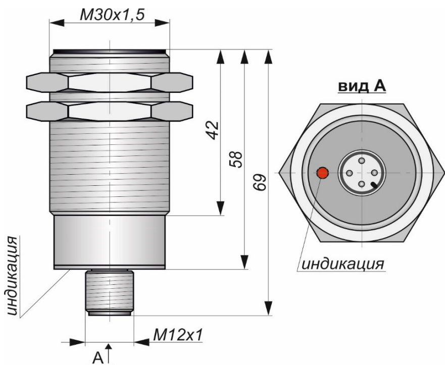
Габаритный чертеж
