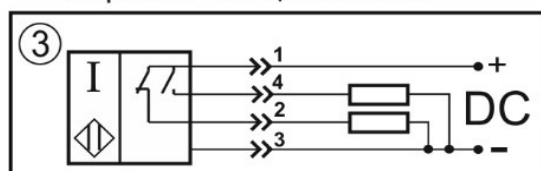
Переключающий контакт
