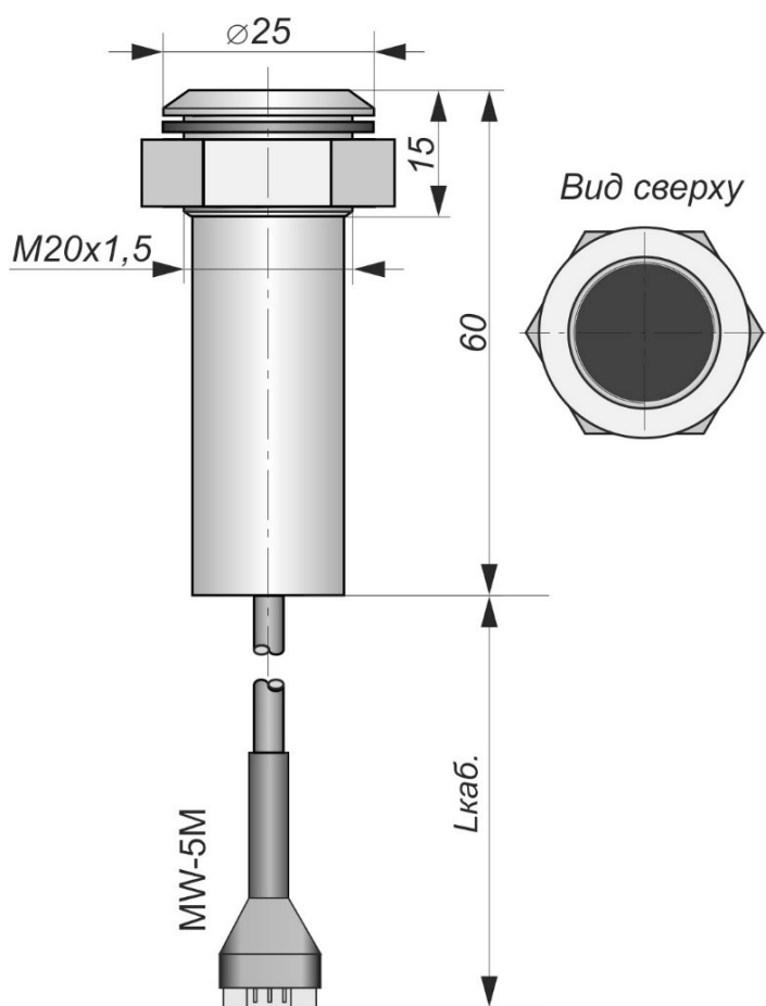
Габаритный чертеж
