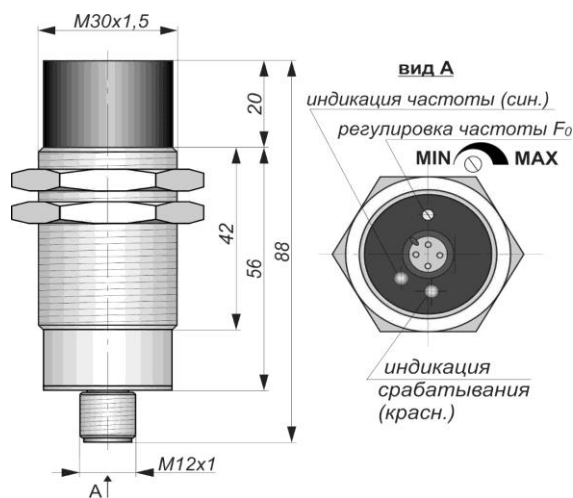
Габаритный чертеж
