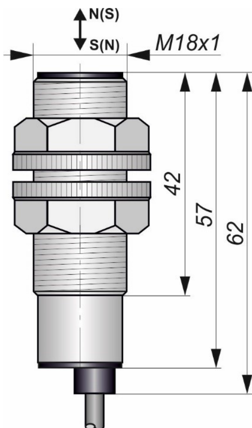
Габаритный чертеж
