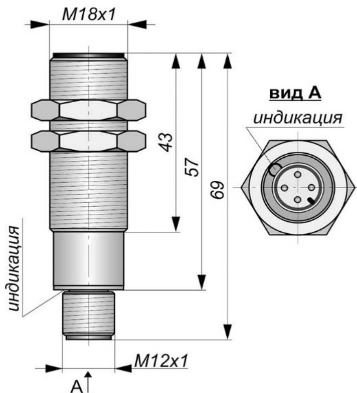
Габаритный чертеж
