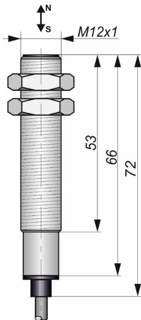
Габаритный чертеж
