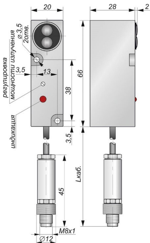
Габаритный чертеж
