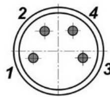
Цоколевка разъема
