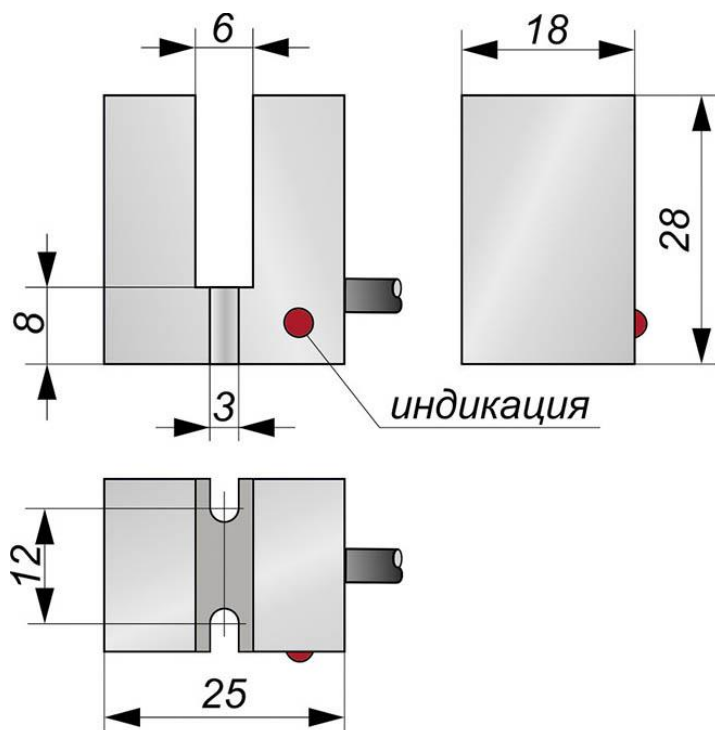
Габаритный чертеж
