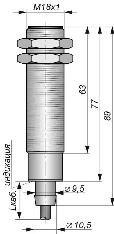
Габаритный чертеж
