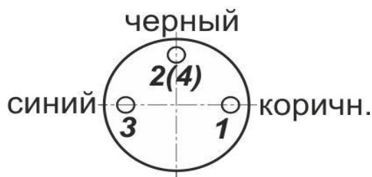
цоколевка разъема
