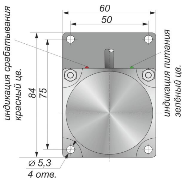
Габаритный чертеж
