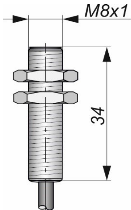
Габаритный чертеж
