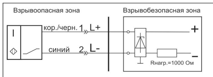
Схема соединения
