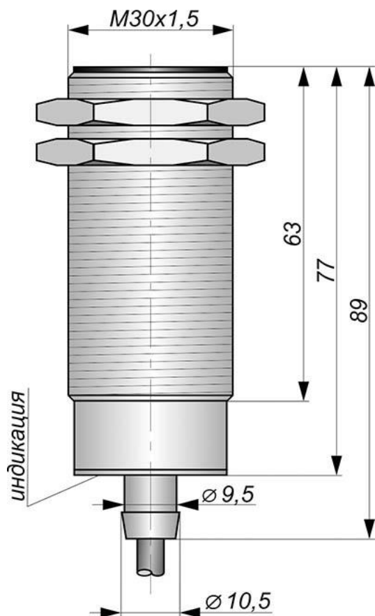
Габаритный чертеж
