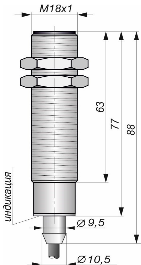
Габаритный чертеж
