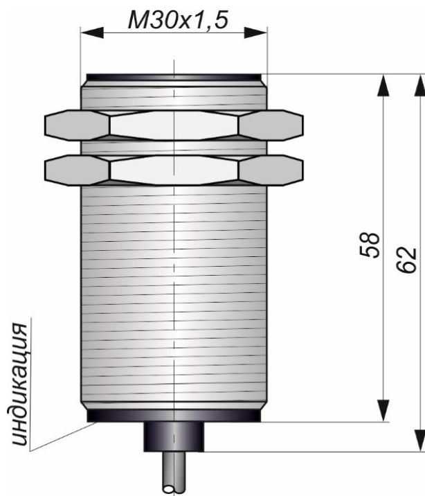
Габаритный чертеж
