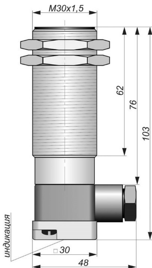
Габаритный чертеж
