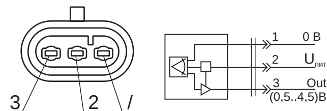
Цоколевка разъема
