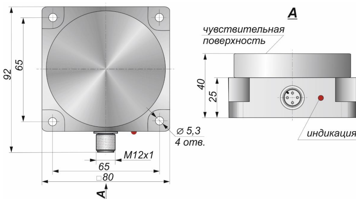
Габаритный чертеж
