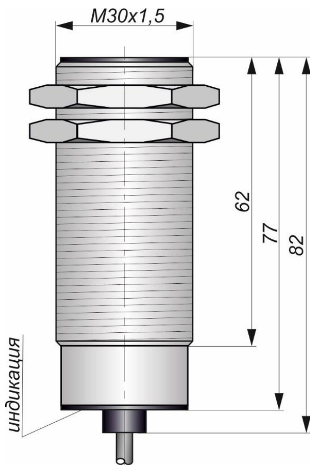
Габаритный чертеж
