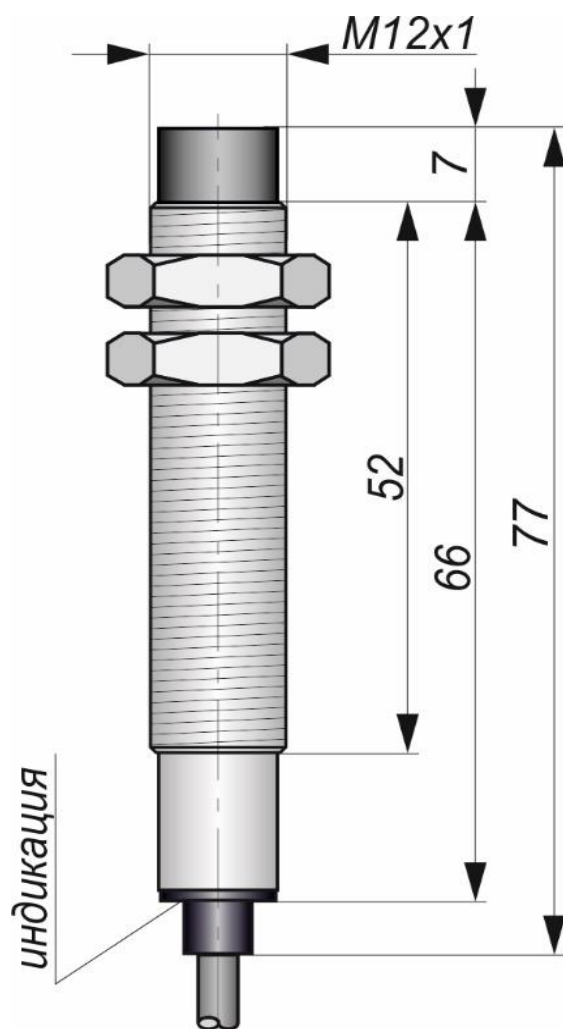
Габаритный чертеж
