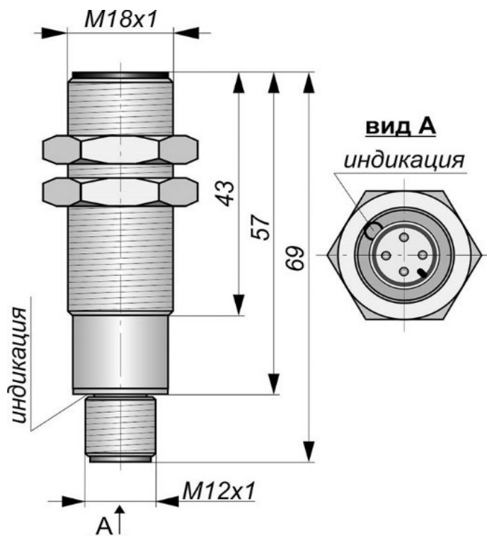
Габаритный чертеж
