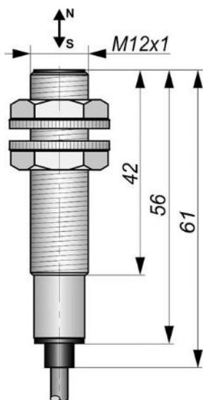
Габаритный чертеж
