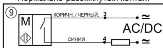
Схема соединения
