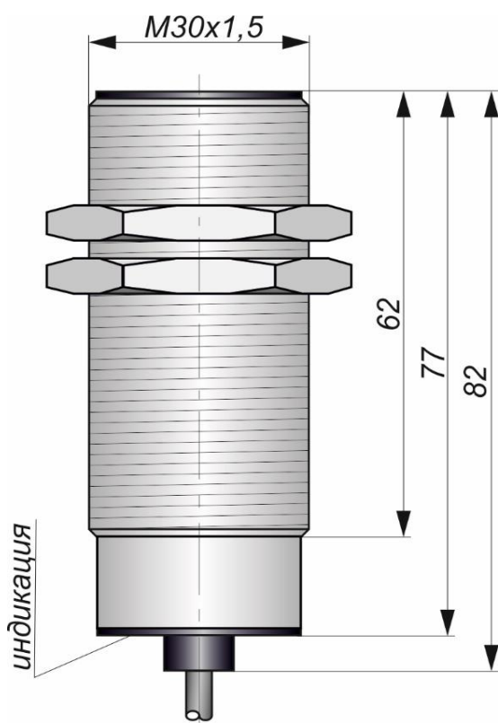
Габаритный чертеж
