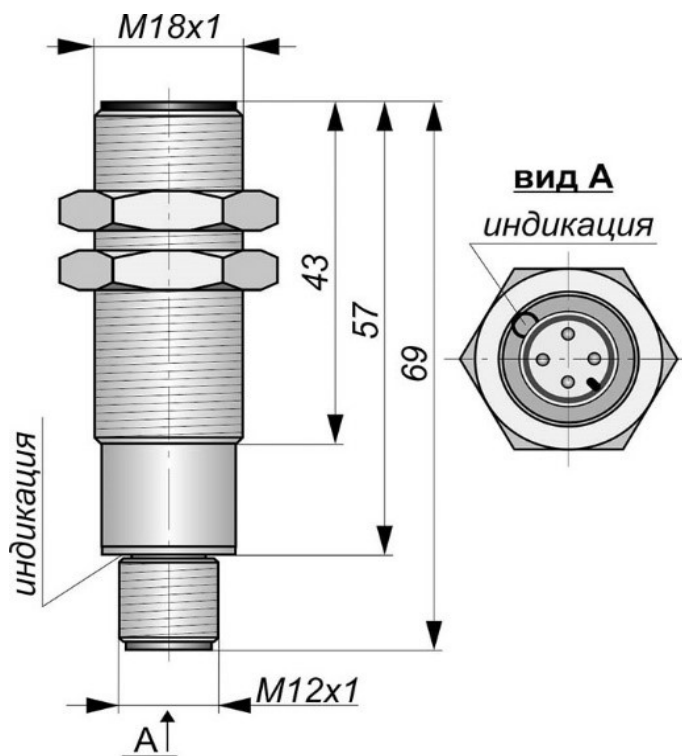
Габаритный чертеж
