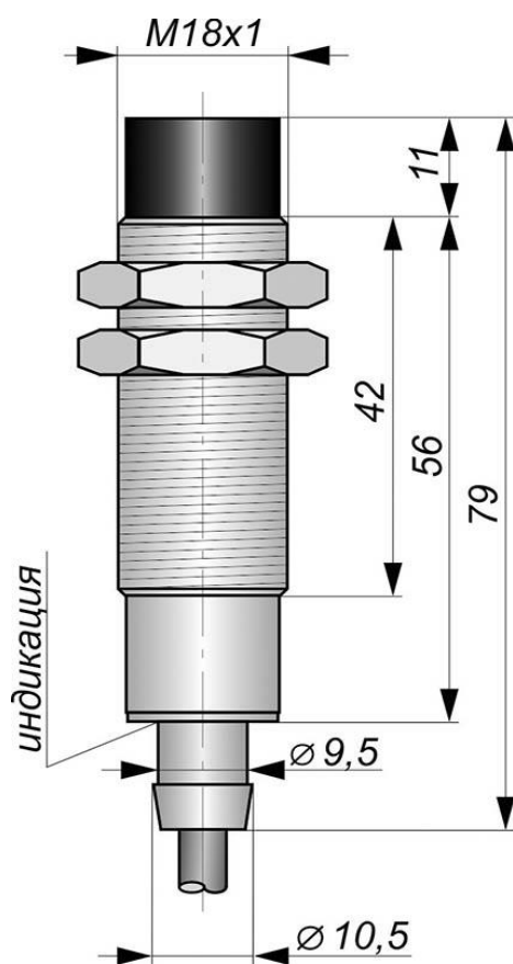
Габаритный чертеж
