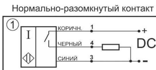
Схема соединения
