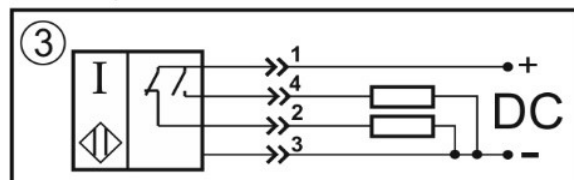
Переключающий контакт
