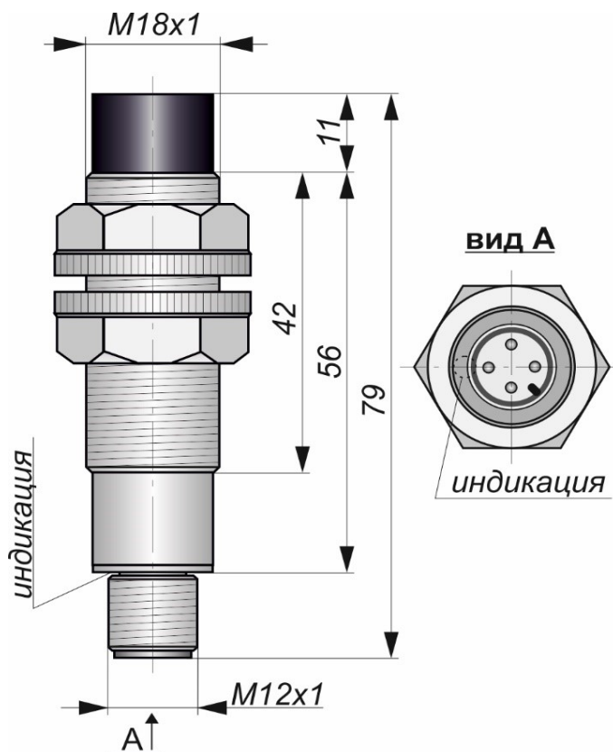
Габаритный чертеж
