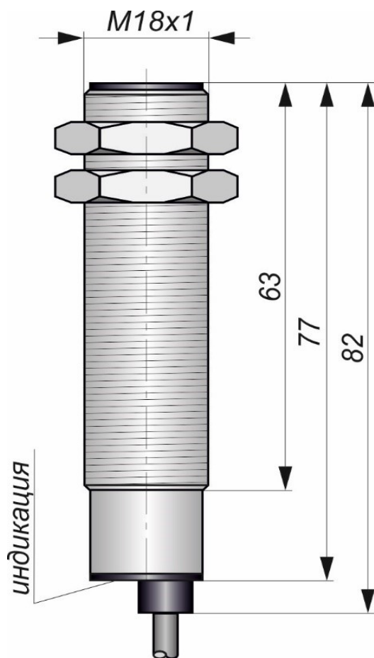
Габаритный чертеж
