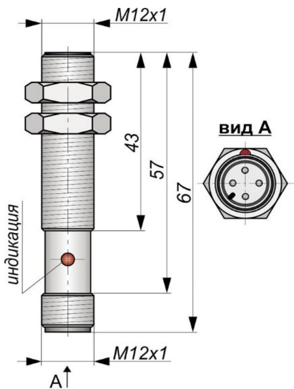
Габаритный чертеж
