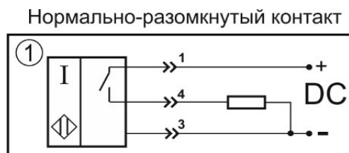
Схема соединения
