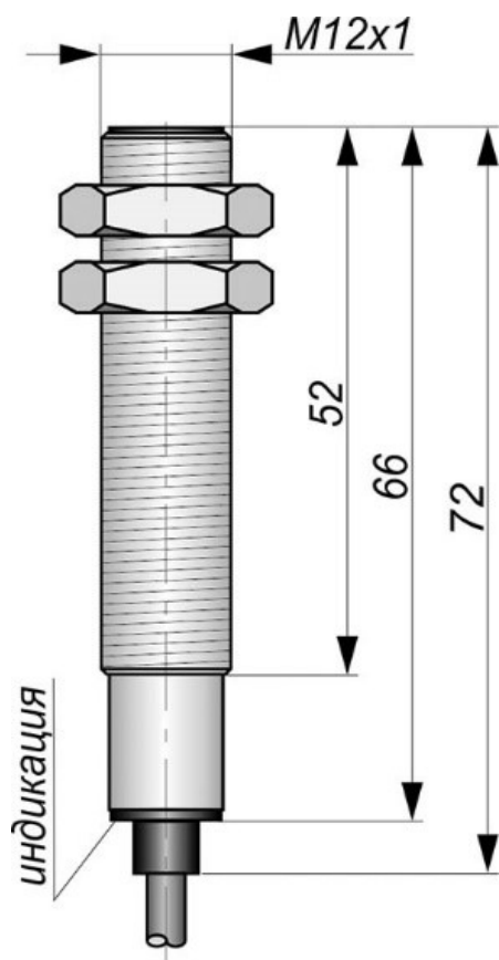
Габаритный чертеж
