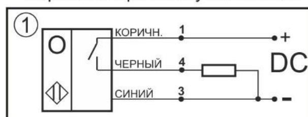
Цоколевка разъема
