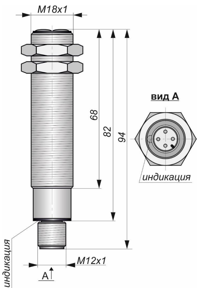
Габаритный чертеж
