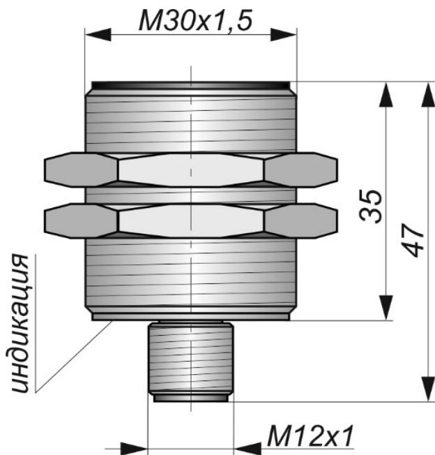
Габаритный чертеж
