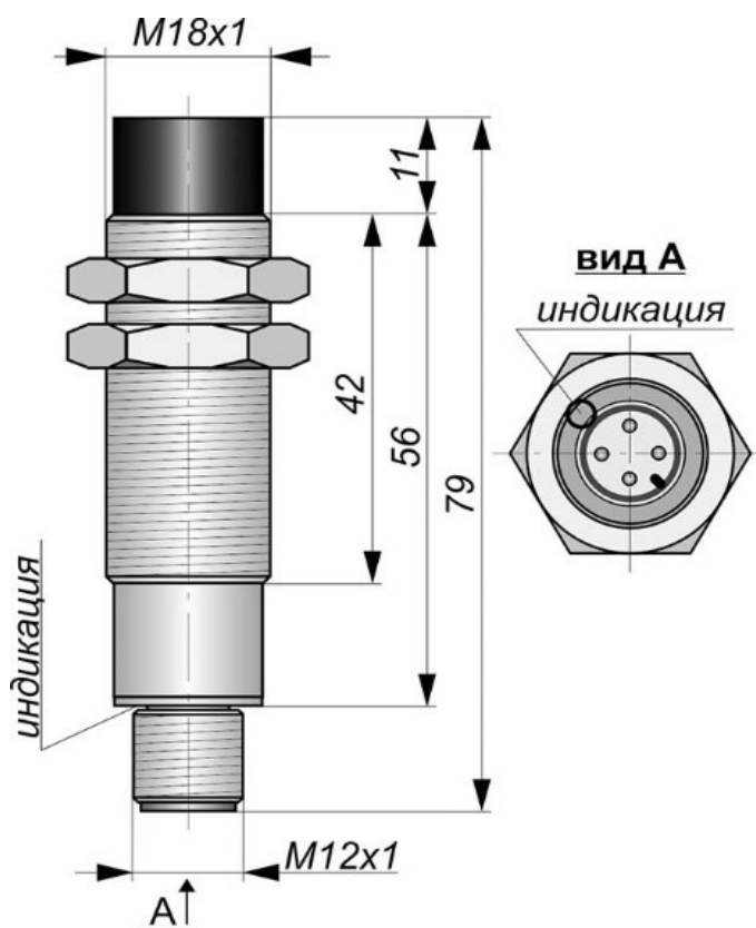
Габаритный чертеж
