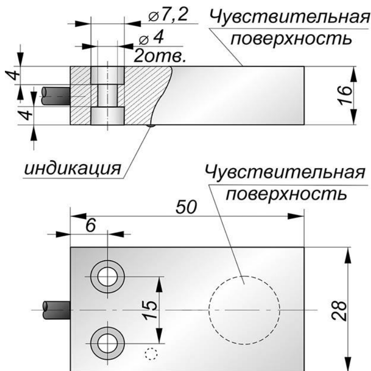
Габаритный чертеж
