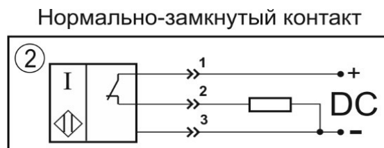
Схема соединения
