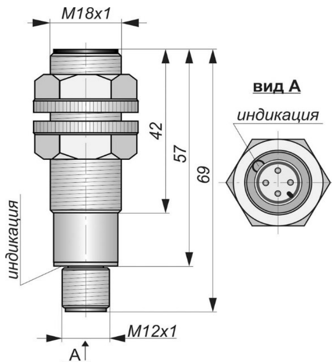
Габаритный чертеж
